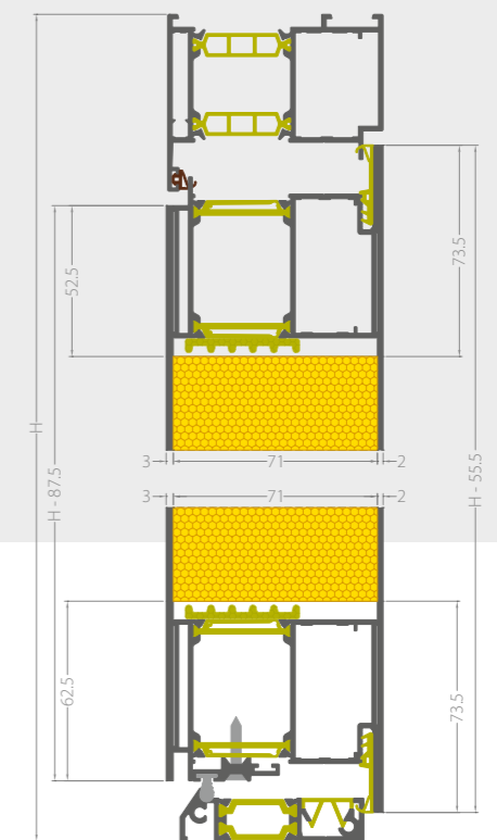
Querschnitt des Türrahmens mit einer Stärke von 75 mm. Füllung mit einer Stärke von 76 mm.
