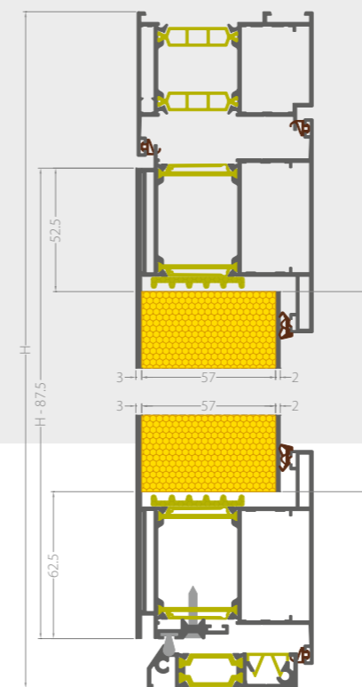
Querschnitt des Türrahmens mit einer Stärke von 75 mm. Füllung mit einer Stärke von 62 mm.
